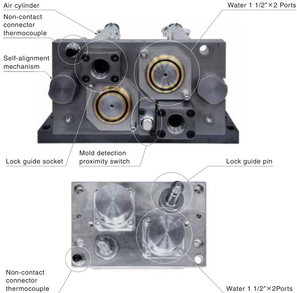
Die side width : 280 × height : 180 (mm)
